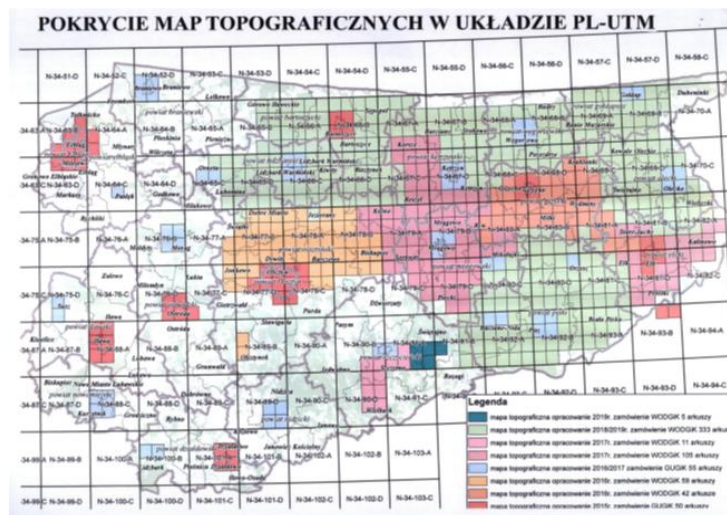
Mapa 3. Pokrycie map topograficznych w układzie PL-UTM
